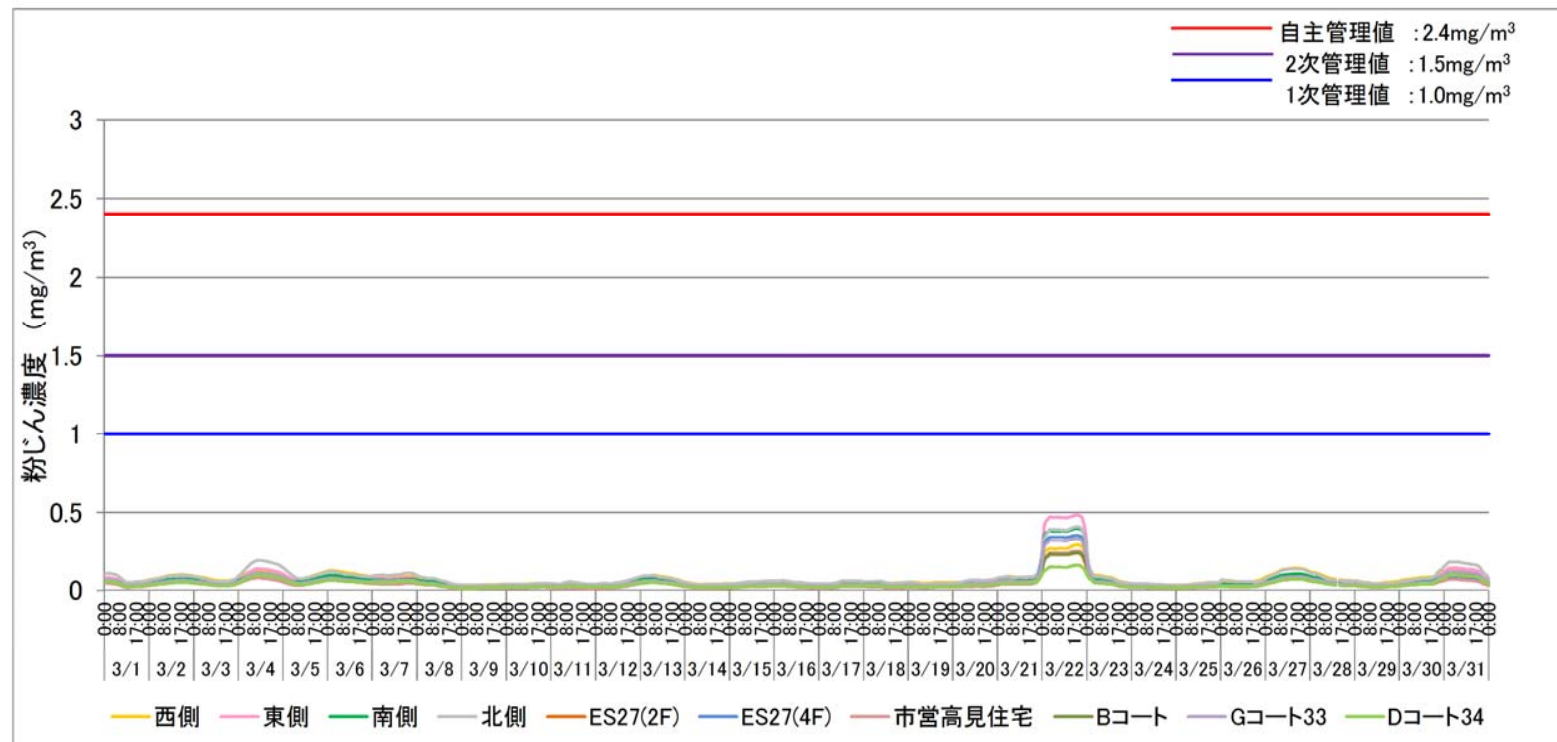
2019.3月度 粉じん濃度24時間移動平均値 (○:管理値超過なし、■:1次管理値超過、▲:2次管理値超過、×:自主管理値超過、-:データの欠測)
