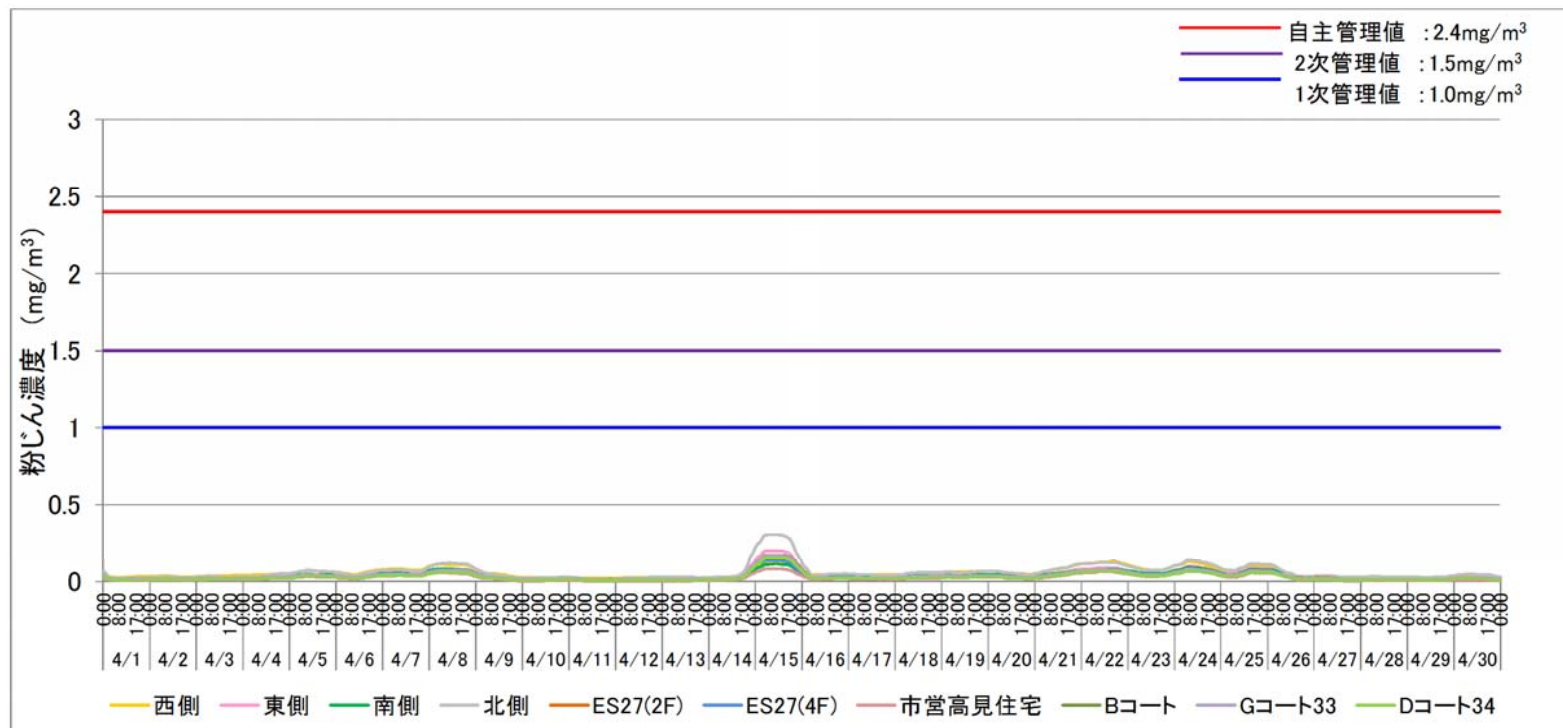
2019.4月度 粉じん濃度24時間移動平均値 (○:管理値超過なし、■:1次管理値超過、▲:2次管理値超過、×:自主管理値超過、-:データの欠測)
