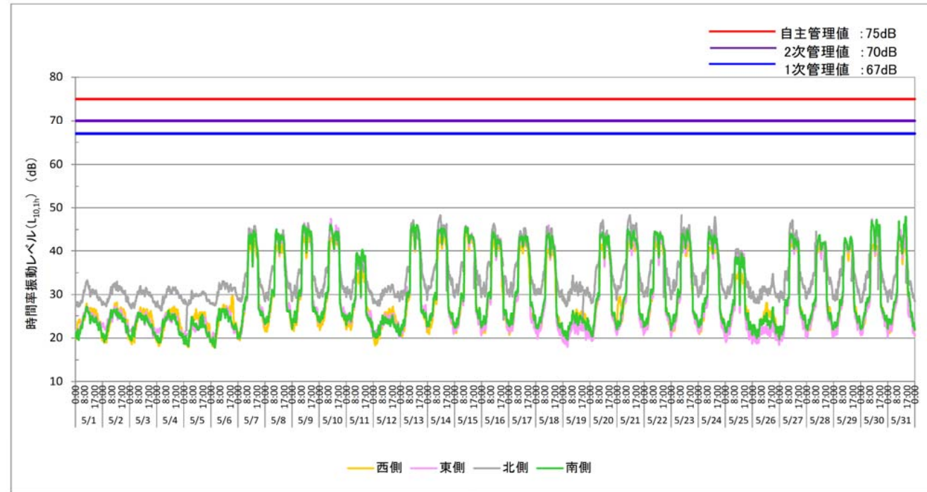
2019.5月度 時間率振動レベル L_{10,1h} (○:管理値超過なし、■:1次管理値超過、▲:2次管理値超過、×:自主管理値超過、-:データの欠測)
