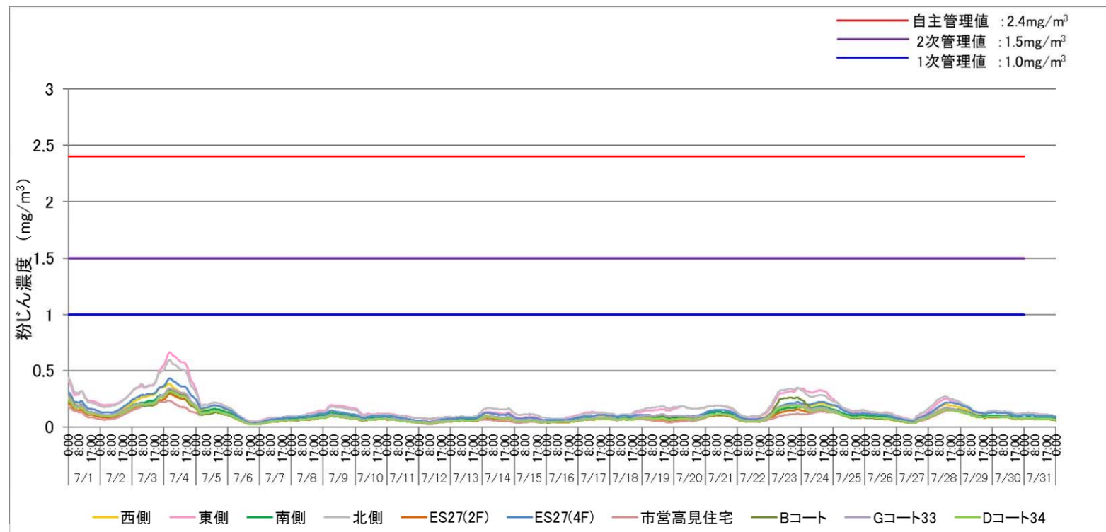
2019.7月度 粉じん濃度24時間移動平均値 (○:管理値超過なし、■:1次管理値超過、▲:2次管理値超過、×:自主管理値超過、-:データの欠測)
