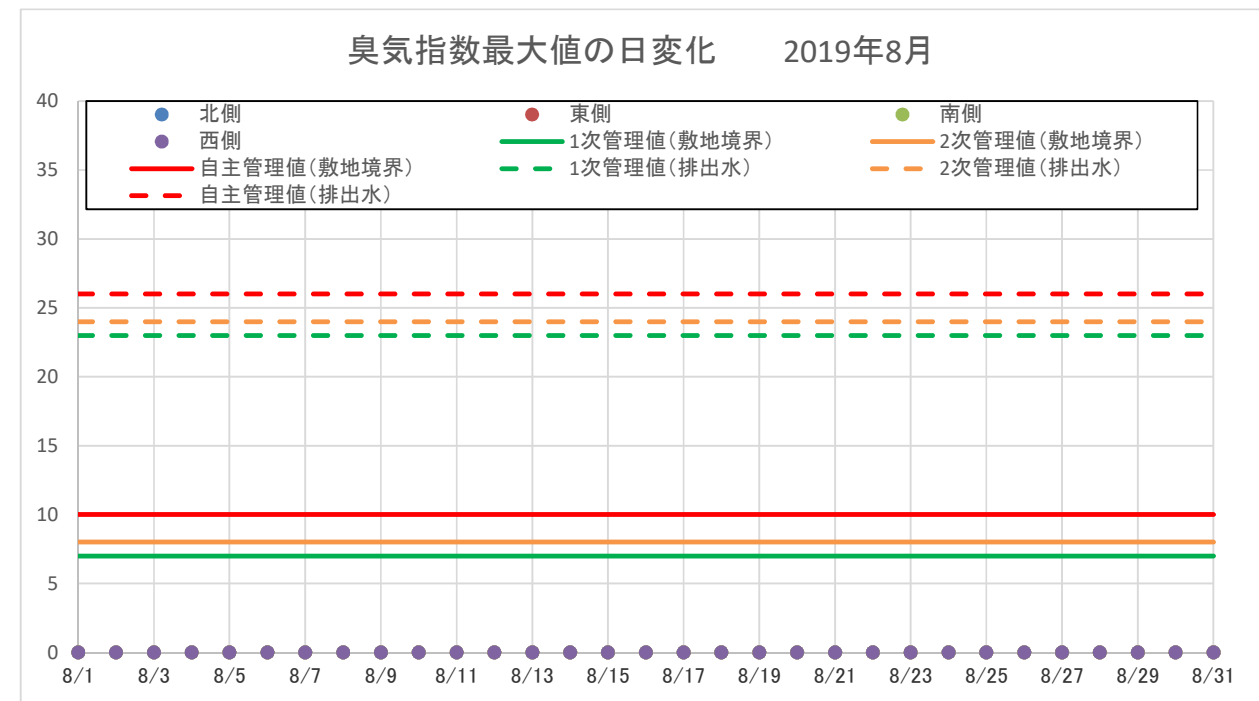
2019.8月度 臭気指数 (○：管理値超過なし、■：1次管理値超過、▲：2次管理値超過、×：自主管理値超過、-：データの欠測)
