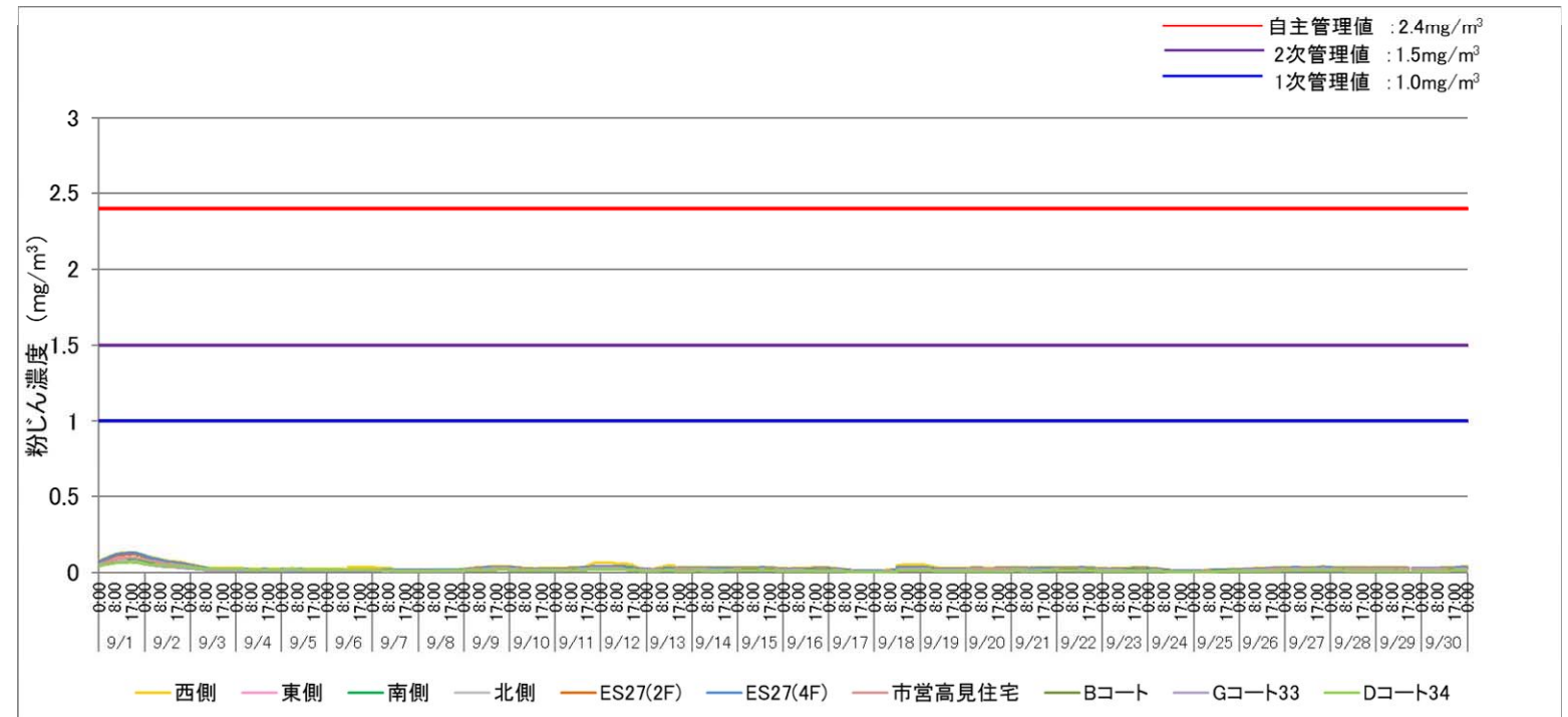
2019.9月度 粉じん濃度24時間移動平均値 (○:管理値超過なし、■:1次管理値超過、▲:2次管理値超過、×:自主管理値超過、-:データの欠測)
