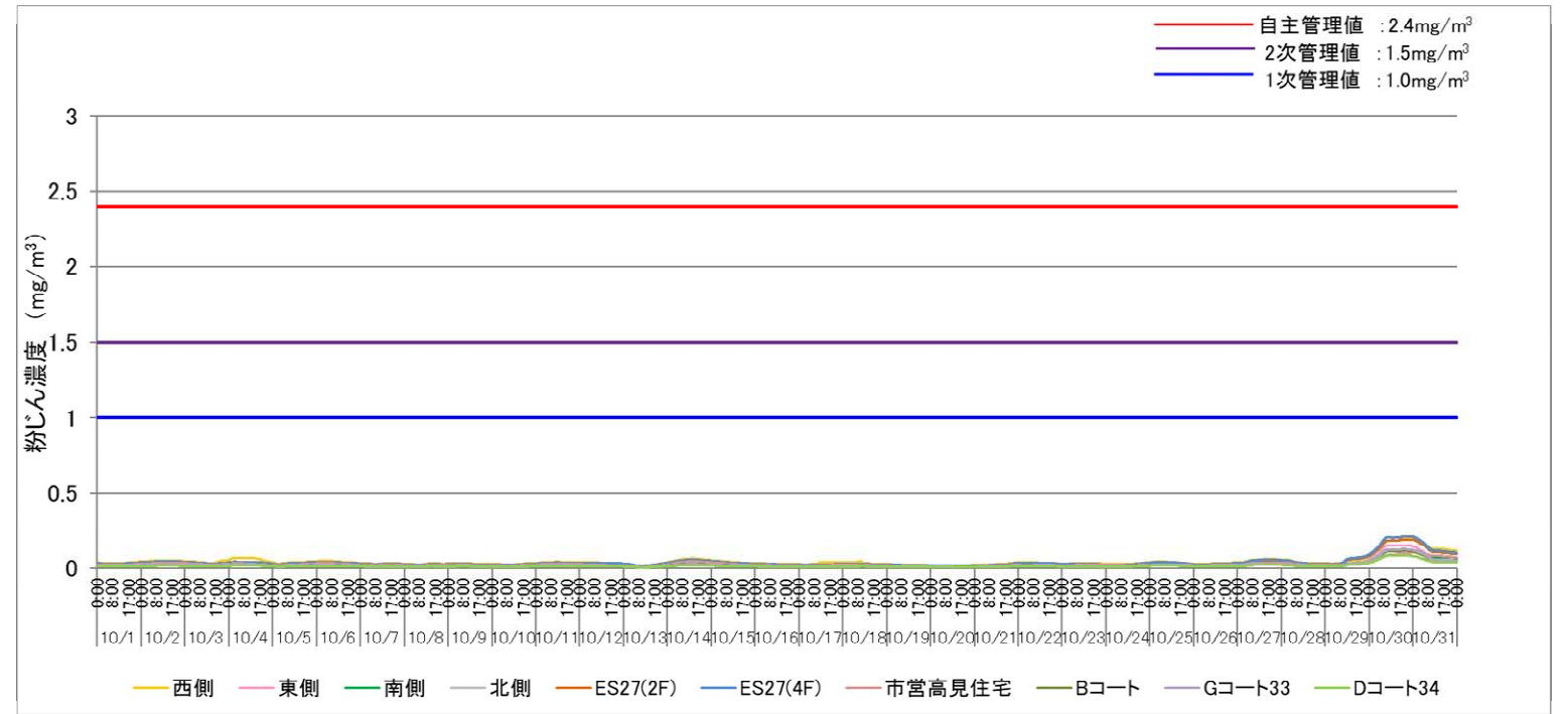
2019.10月度 粉じん濃度24時間移動平均値 (○：管理値超過なし、■：1次管理値超過、▲：2次管理値超過、×：自主管理値超過、-：データの欠測)
