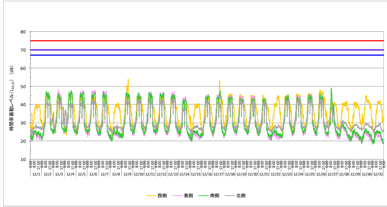
2019.12月度 時間率振動レベル L_{10,1h} (○:管理値超過なし、■:1次管理値超過、▲:2次管理値超過、×:自主管理値超過、-:データの欠測)
