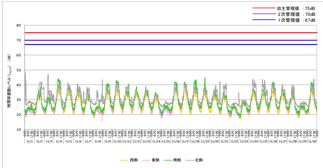
2020.11月度 時間率振動レベル L_{10,1h} (○:管理値超過なし、■:1次管理値超過、▲:2次管理値超過、×:自主管理値超過、-:データの欠測)
