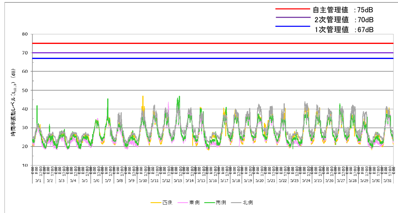
2021.5月度 時間率振動レベル L_{10,1h} (○：管理値超過なし、■：1次管理値超過、▲：2次管理値超過、×：自主管理値超過、-：データの欠測)
