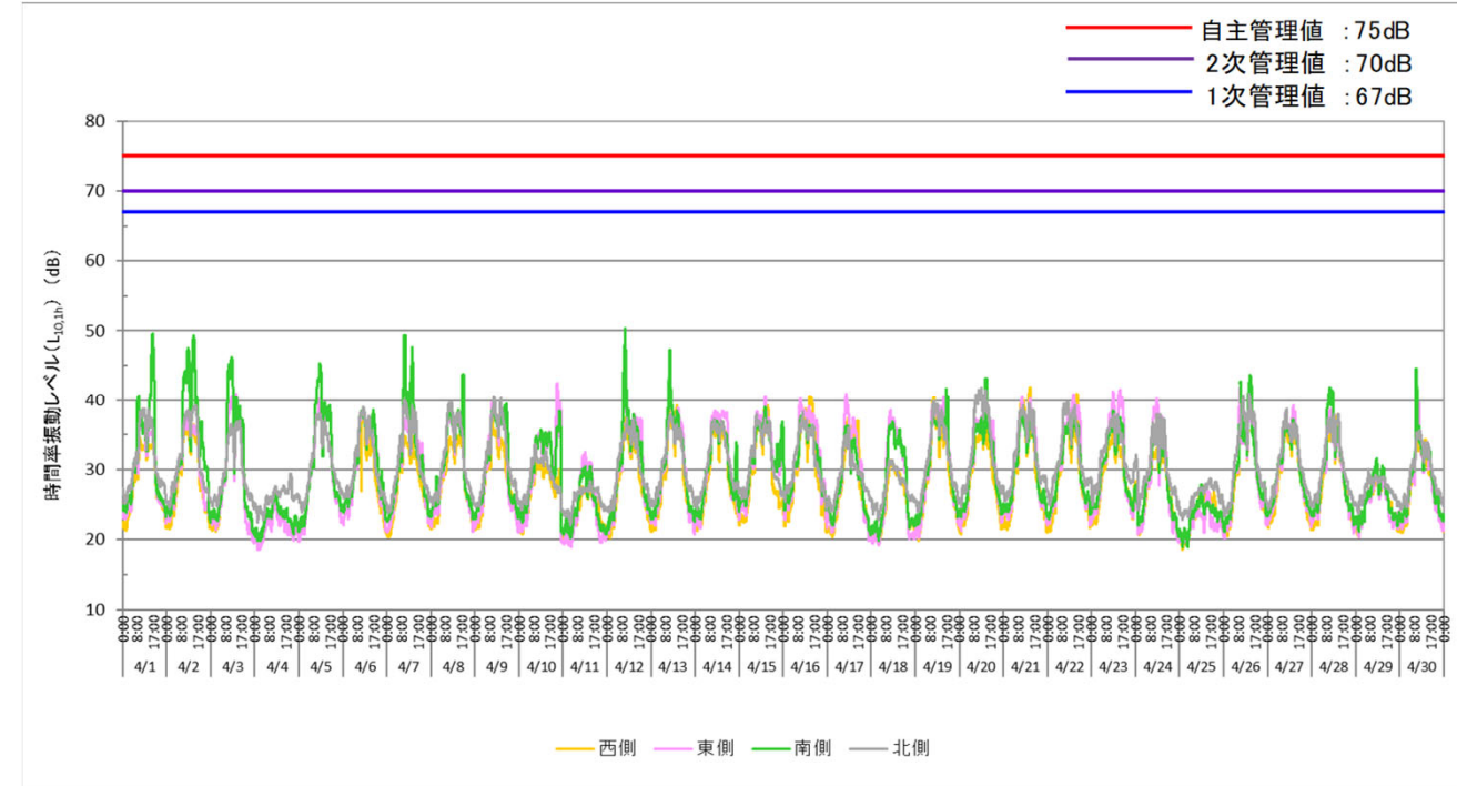
2021.4月度 時間率振動レベル L_{10,1h} (○：管理値超過なし、■：1次管理値超過、▲：2次管理値超過、×：自主管理値超過、-：データの欠測)
