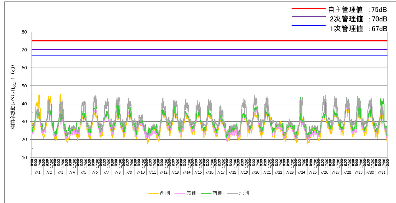
2021.7月度 時間率振動レベル L_{10,1h} (○：管理値超過なし、■：1次管理値超過、▲：2次管理値超過、×：自主管理値超過、-：データの欠測)
