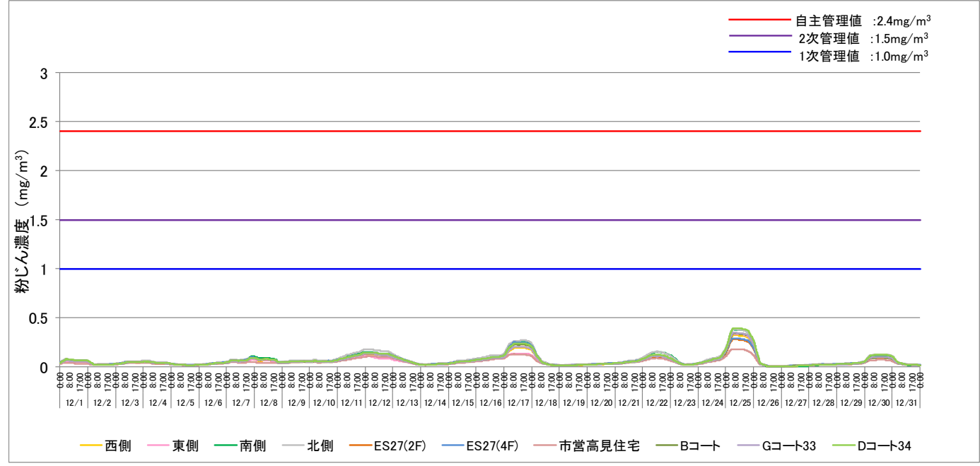
2021.12月度 粉じん濃度24時間移動平均値 (○：管理値超過なし、■：1次管理値超過、▲：2次管理値超過、×：自主管理値超過、-：データの欠測)
