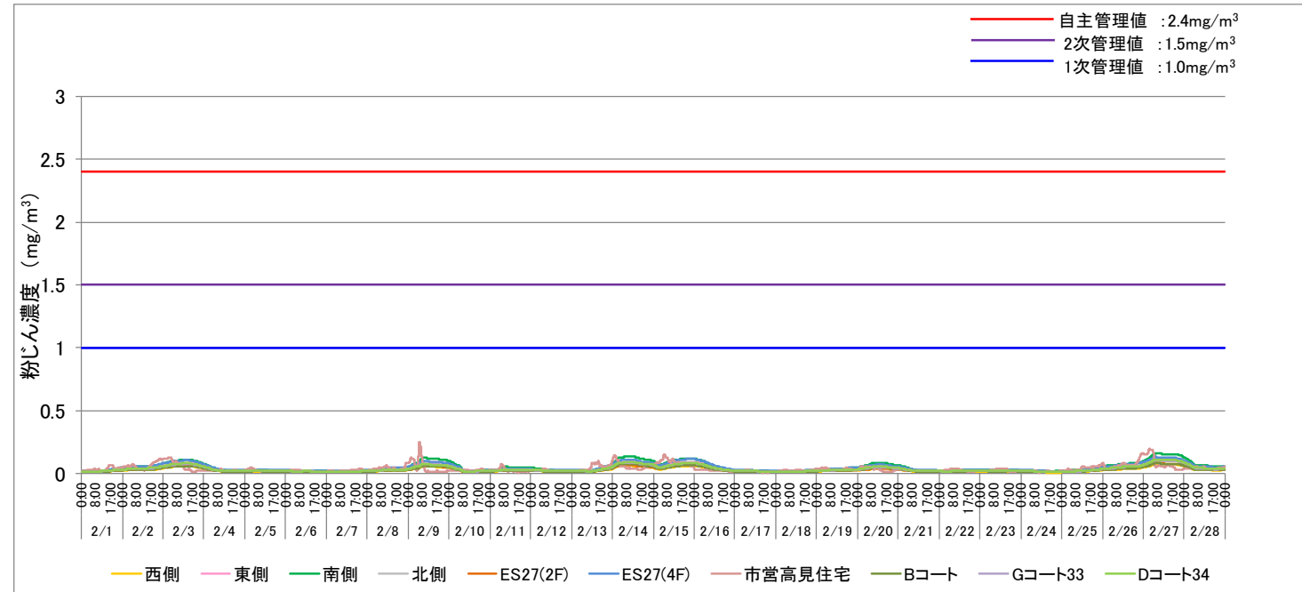
2022.2月度 粉じん濃度24時間移動平均値 (○：管理値超過なし、■：1次管理値超過、▲：2次管理値超過、×：自主管理値超過、-：データの欠測) 単位：mg/m 3
