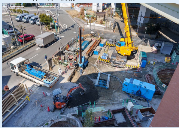
・ポンプ棟立坑：開削工
