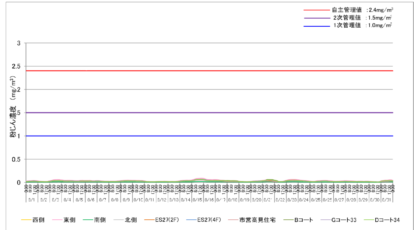
2022.8月度 粉じん濃度24時間移動平均値 (○：管理値超過なし、■：1次管理値超過、▲：2次管理値超過、×：自主管理値超過、-：データの欠測)
