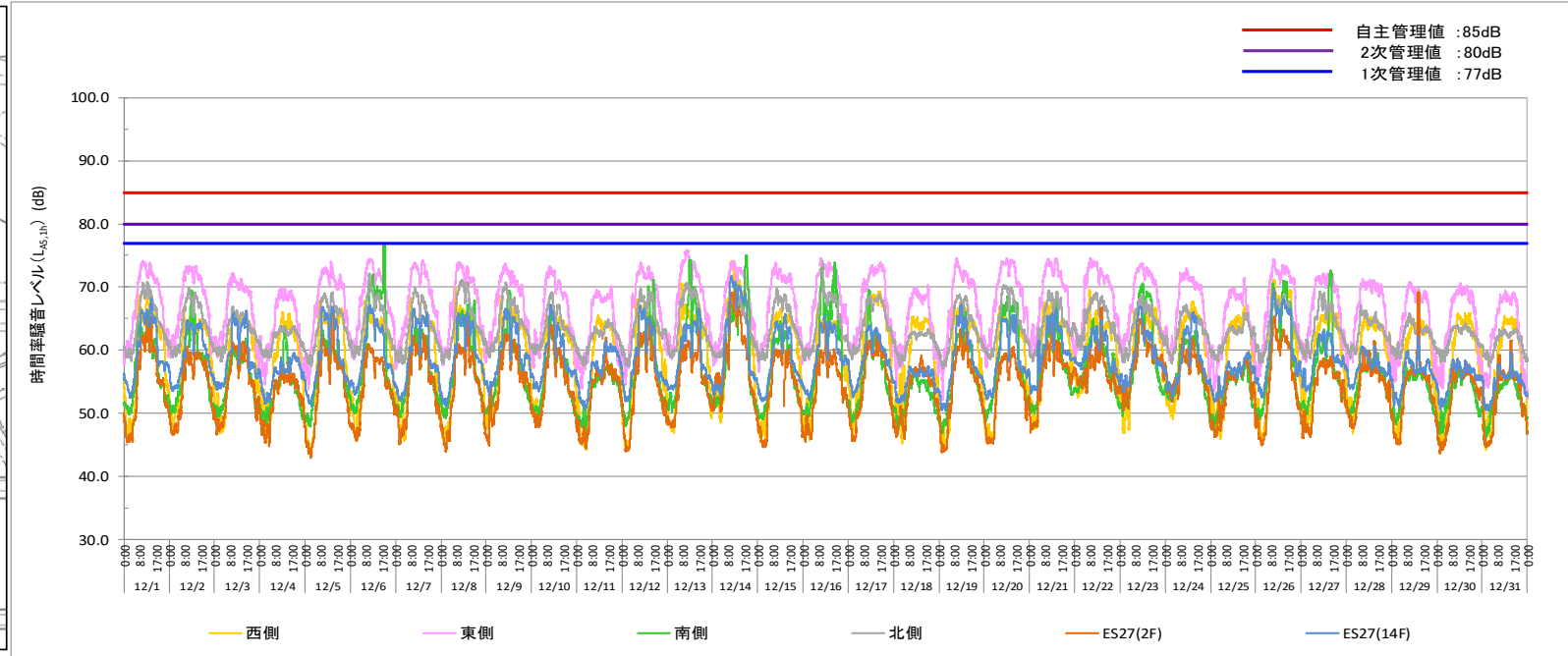
2022.12月度 時間率騒音レベルLA5,1h (○:管理値超過なし、■:1次管理値超過、▲:2次管理値超過、×:自主管理値超過、-:データの欠測)
