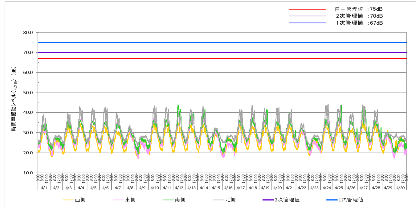
2023.4月度 時間率振動レベルL10, 1h (○: 管理値超過なし、■: 1次管理値超過、▲: 2次管理値超過、×: 自主管理値超過、-: データの欠測)
