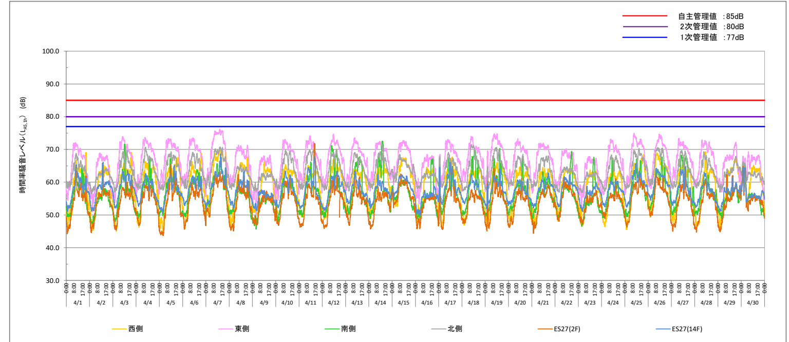
2023.4月度 時間率騒音レベルLA5,1h (○：管理値超過なし、■：1次管理値超過、▲：2次管理値超過、×：自主管理値超過、-：データの欠測)
