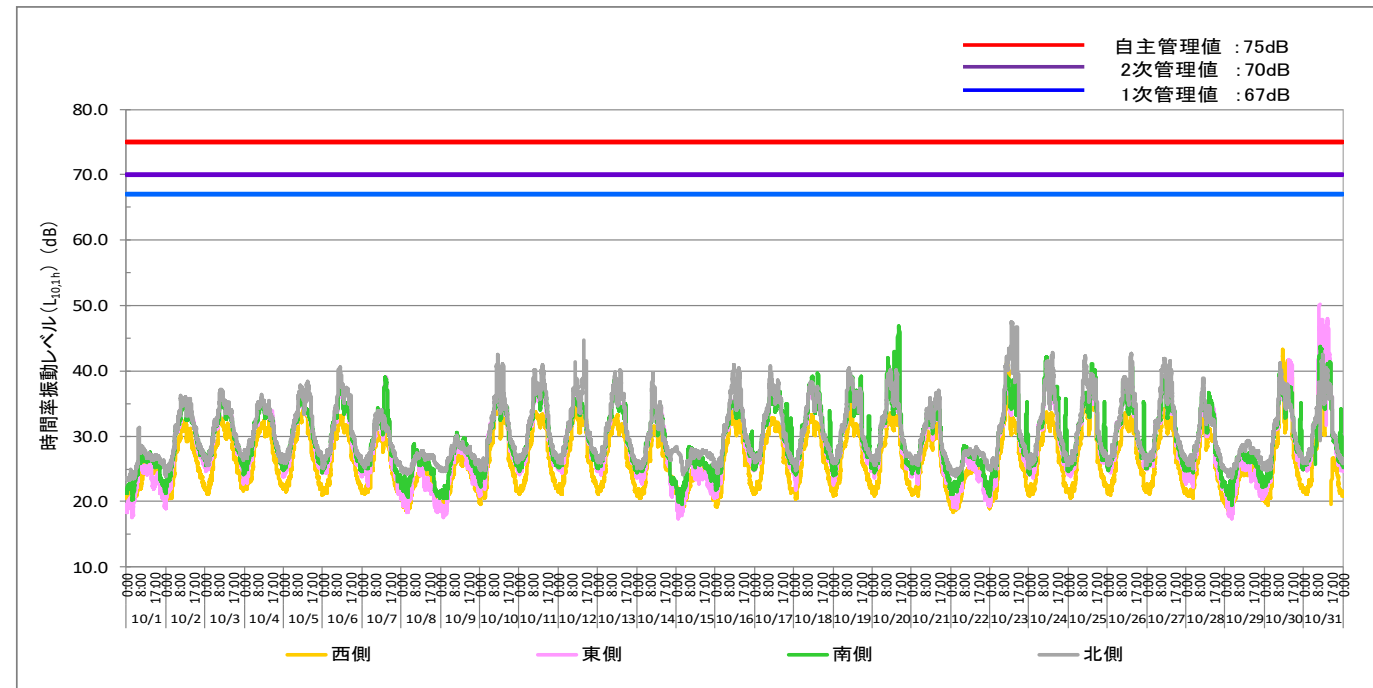
2023.10月度 時間率振動レベルL10,1h (○:管理値超過なし、■:1次管理値超過、▲:2次管理値超過、×:自主管理値超過、-:データの欠測)
