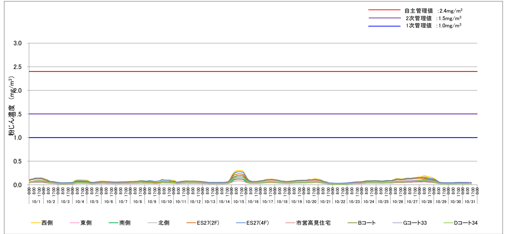
2023.10月度 粉じん濃度24時間移動平均値 (○:管理値超過なし、■:1次管理値超過、▲:2次管理値超過、×:自主管理値超過、-:データの欠測)
