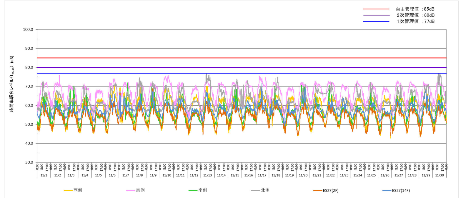
2023.11月度 時間率騒音レベルLA5,1h (○:管理値超過なし、■:1次管理値超過、▲:2次管理値超過、×:自主管理値超過、-:データの欠測)
